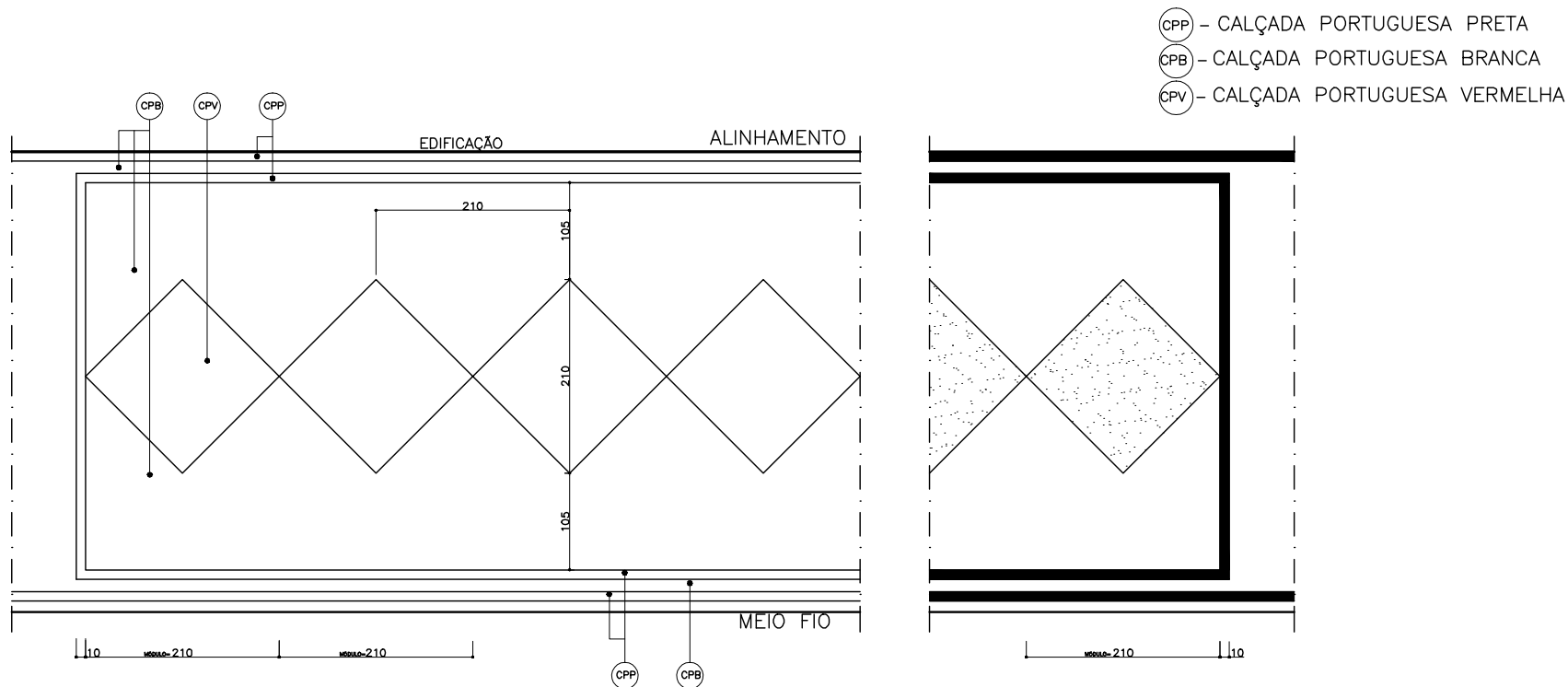
PLANTA – DETALHE PASSEIO AVENIDA AFONSO PENA ESCALA 1/75
