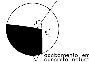
DEGRAU. DET. A ESC1:7,5
