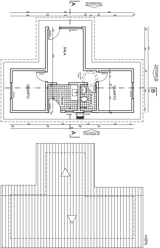
PLANTA 2 QUARTOS - VERSÃO 06 ESCALA..... 1/150
